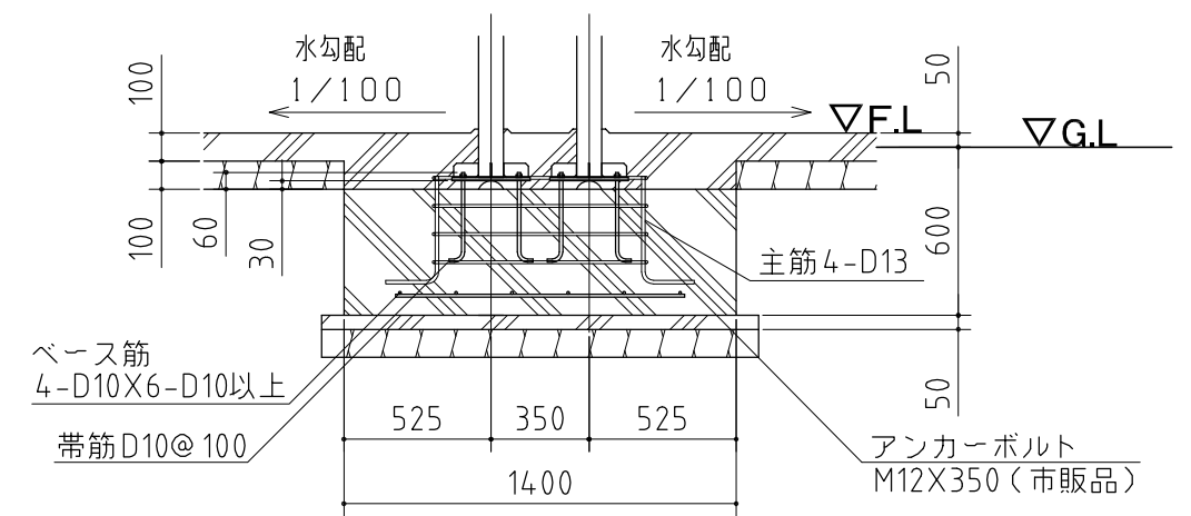
A-A' 断面
